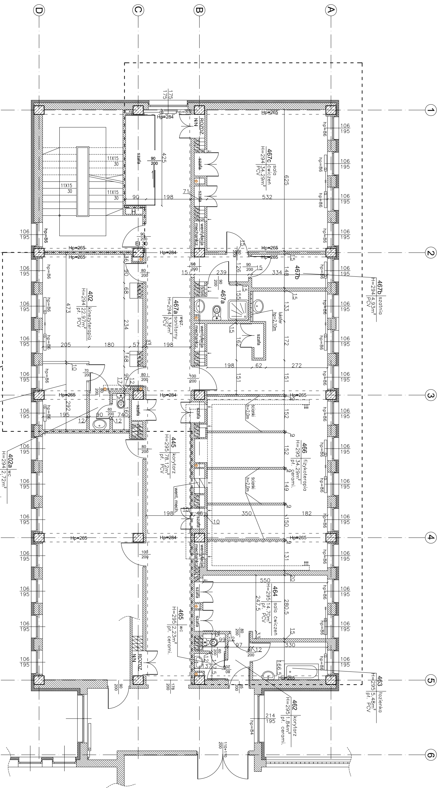
ZESTAWIENIE POWIERZCHNI UŻYTKOWEJ_4 piętro (w zakresie opracowania)
